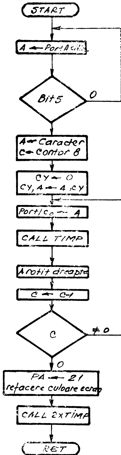
Fig. 6.3. Ordinograma programului de comandă la transmisia serie SERIE.
