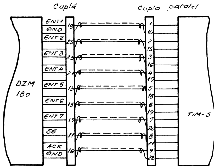
Fig. 4.2.1. Semnale de dialog la TIM-S.
